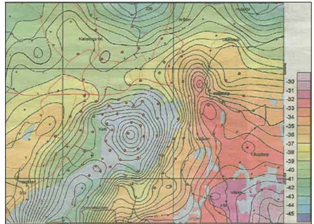
Tyngdkraftsvariationen inom området. Den blå färgen innebär lägre tyngdkraft än den gula och röda.
