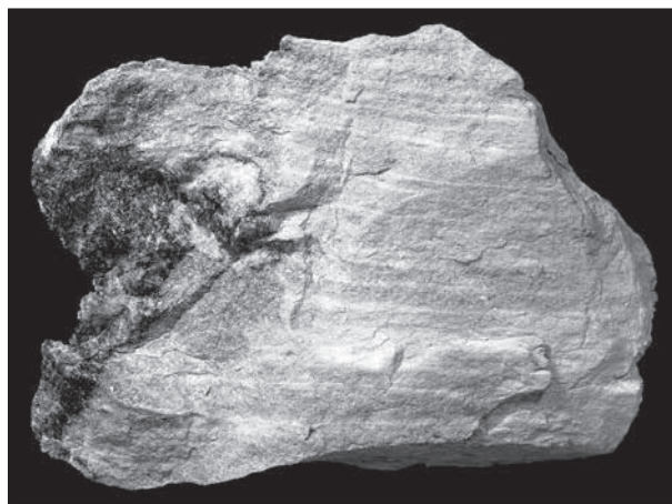
Det finns gott om kyanitkvartsit vid Hålsjöberg, norr om vägen Torsby – Ekshärad.
