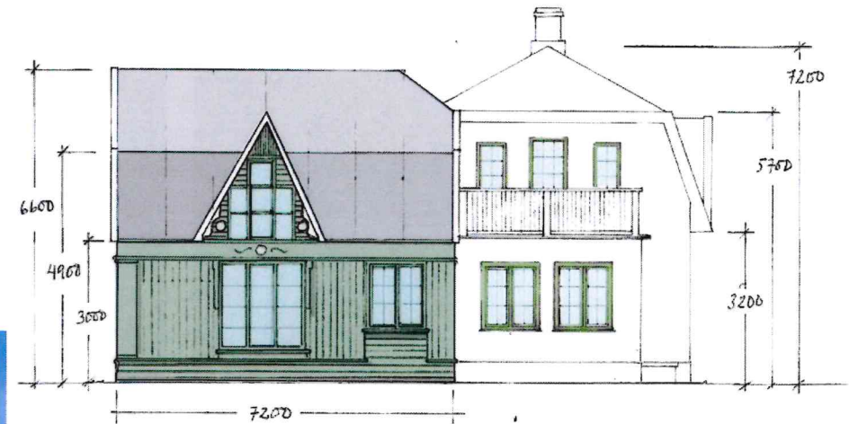
Bygglösningsritning A2 Falsterbo 6:68 - Tillbyggnad
